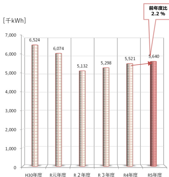
栄谷団地の使用電力量[kWh]の推移 (H30～令和5)
